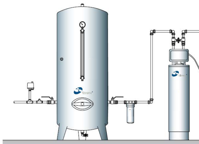
Installationsskiss
